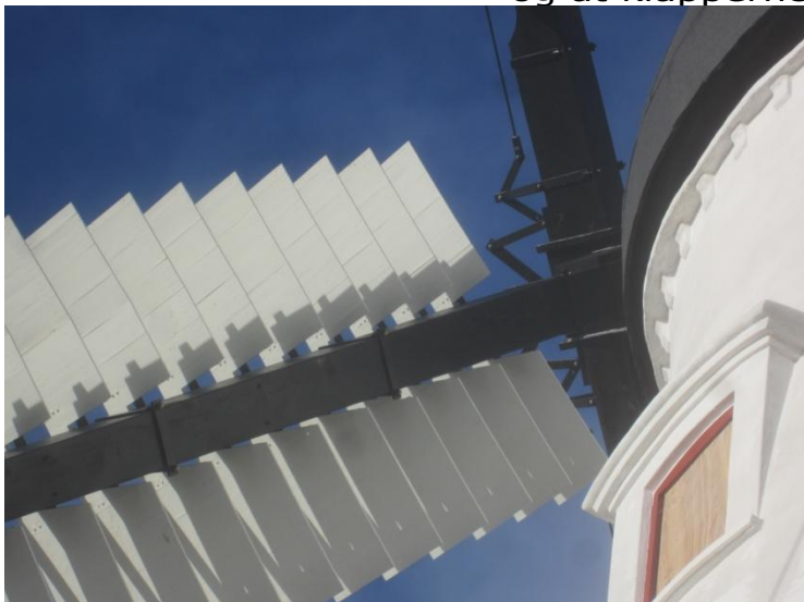
Her ses Edderkoppen der styrer klapperne via kædetræk fra Svikstillingen
