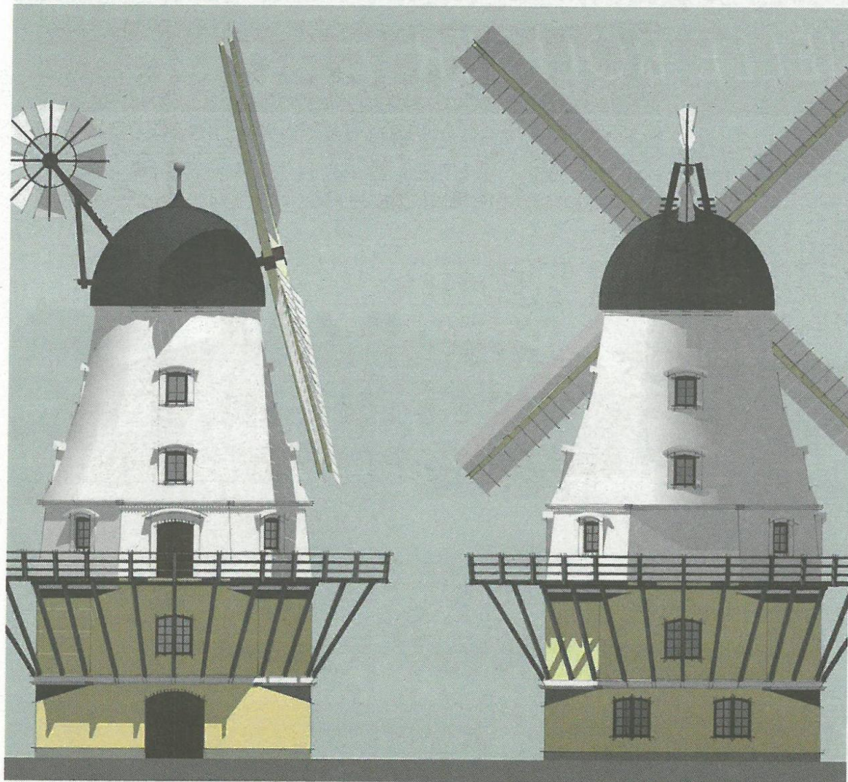
Tegninger af den færdigrenoverede Christiansmøllen.
